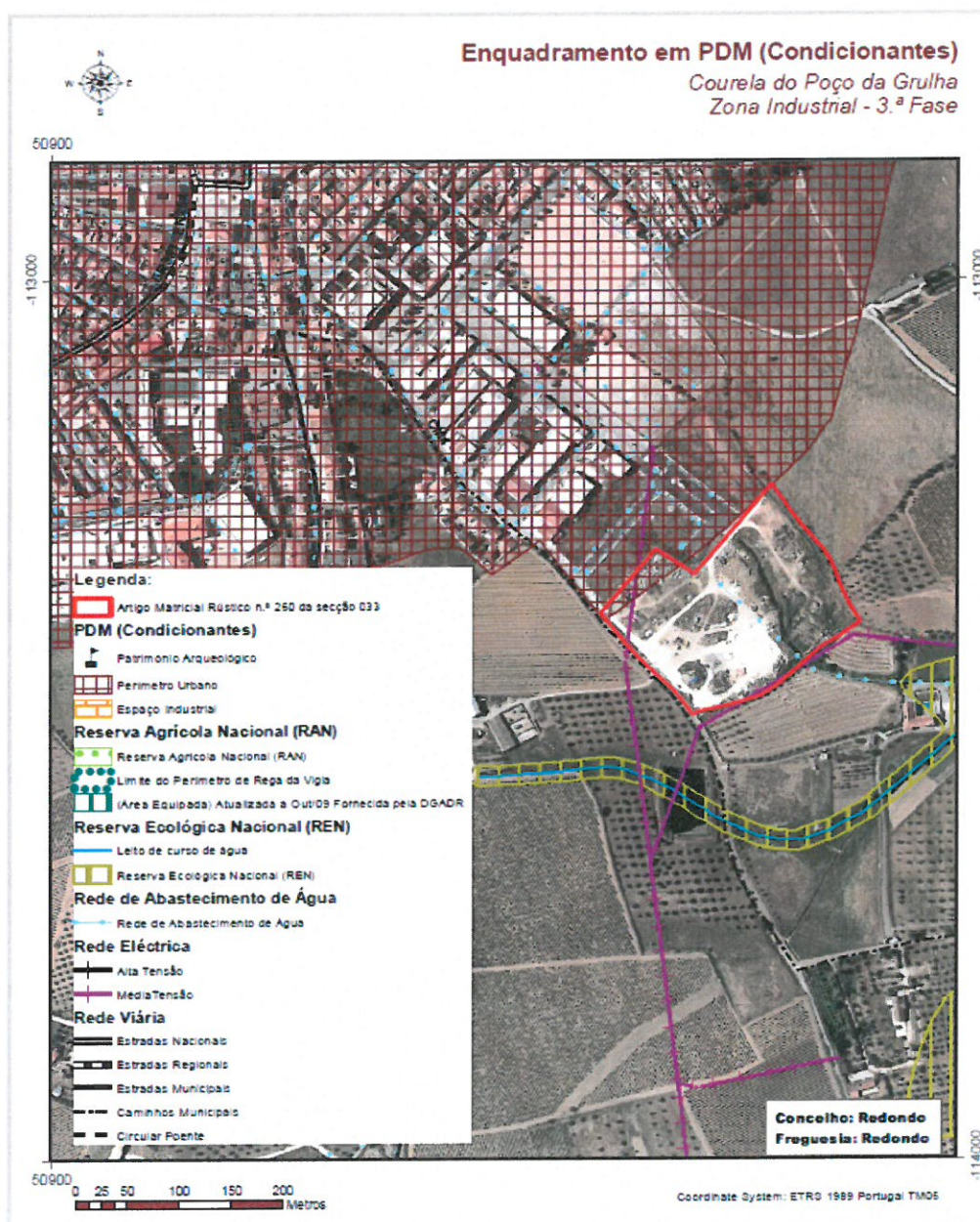
Figura 3 - Planta de Condicionantes da Courela do Poço do Grulha
